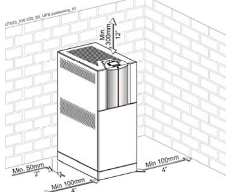
Рис. 5.4-1 Расположение ИБП
