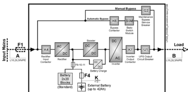
Рис. 5.7.2-2 Общий вход выпрямителя и байпаса
