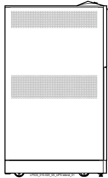
Рис. 2.2-3 Вид сбоку
