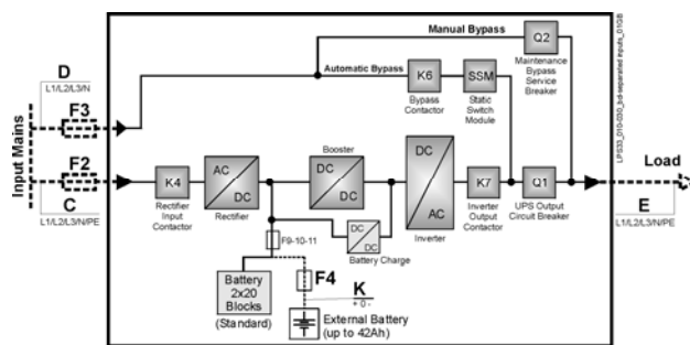
Рис. 5.7.3-2 Раздельный вход выпрямителя и байпаса (опция)
