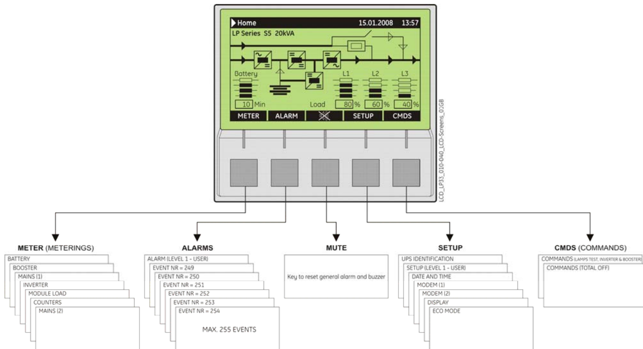
Рис. 7.1-1 ЖК-дисплей
