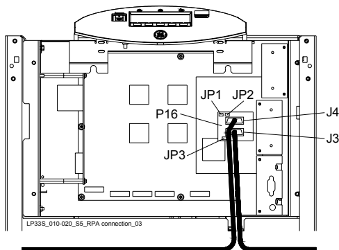
Рис. 5.8.4-3 Подключение к плате P16
